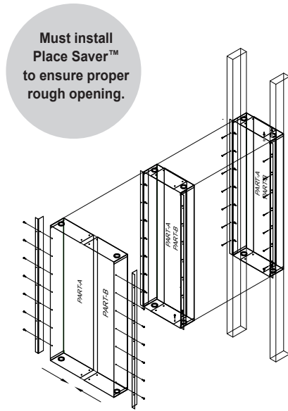
Metal stud / hat channel configuration
